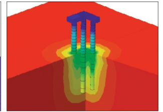
▲ 3차원 기초안정성 검토
