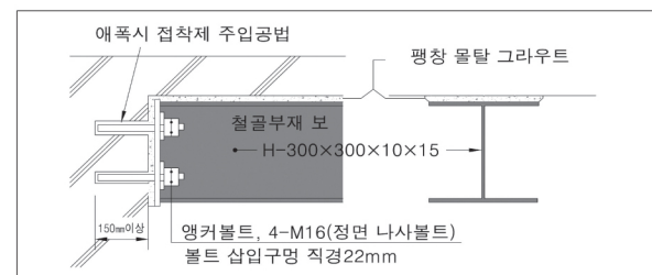
▲ H-BEAM보강 개요도
