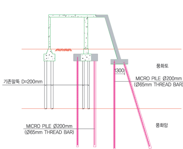
안정성 검토(침하/수평)
