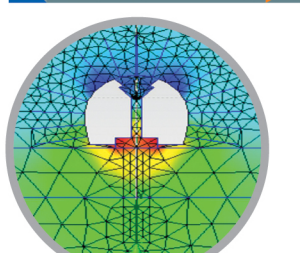
안정성 검토(침하/수평)
