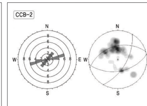
▲ 공내영상촬영
