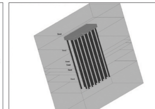
▲ 유사정적해석
