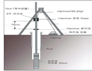
▲ 시추조사 모식도
