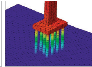
▲ 단층파쇄대 영향검토
