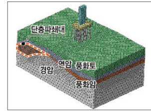
▲ 단층파쇄대 해석모델링
