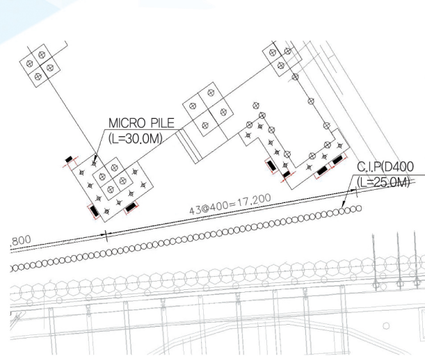
안정성 검토(침하/수평)
