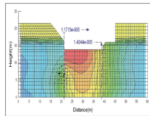
▲ 구조물터파기 침투해석
