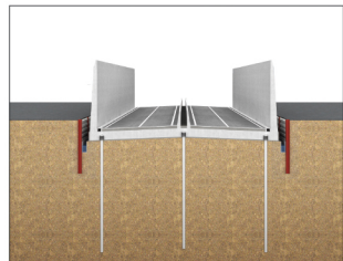
▲ H-PILE 자립검토
