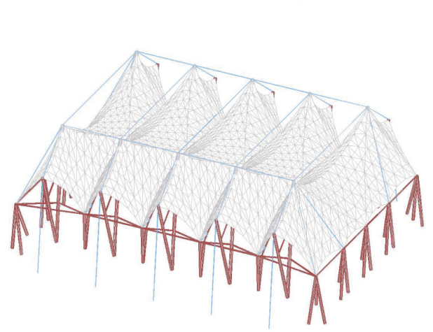
1 강봉 조립
