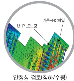
안정성 검토(침하/수평)
