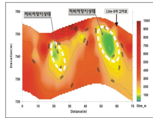
▲ 전기비저항탐사
