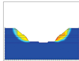
▲ 자연터파기 안정성 검토
