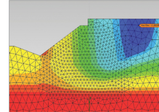
▲ 단층파쇄대 영향검토
