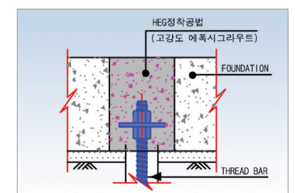
▲ 마이크로파일 상부 두부정착 방법 : 특허 제10-1161844호 (기존기초와 연결시 적용 공법)
