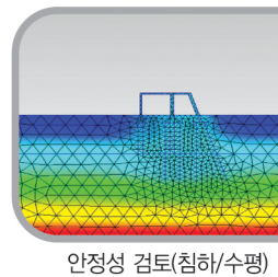
안정성 검토(침하/수평)
